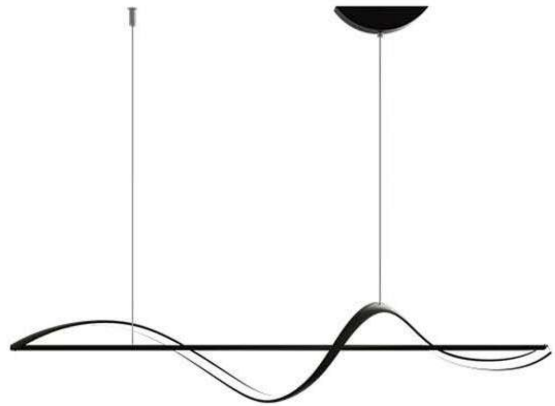
OTMP6694 尺寸/Size : L120*W26cm 功率/Power : LED 36 W 材质/Material : 铝+硅胶/Aluminum+silica gel
